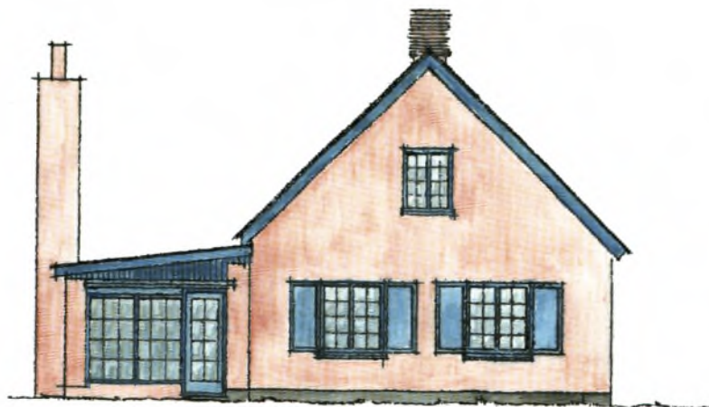
GAVL MOD VEST
