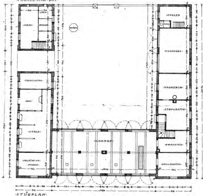
Arkitekt N. Hatting-Jørgensens tegning fra 1919 til Kullabergs garager og stald med domestikboliger i tagetagen (Fredensborg Kommunes Byggesagsarkiv).
