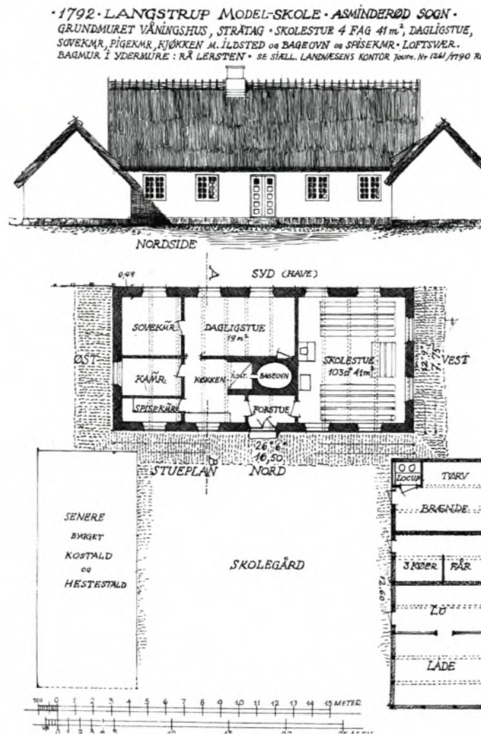
Langstrup skole, Humlebækvej 32 opført efter Adolf von der Reches tegning i 1791 som model for de andre skoler, der blev efter landboreformerne. Grundplan af Langstrup skole
